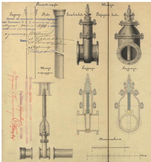
FRAGMENT PROJEKTU TECHNICZNEGO ZAWORÓW ŻELIWNYCH OLKUSKIEGO WODOCIĄGU
